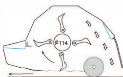
MULS 110-170
